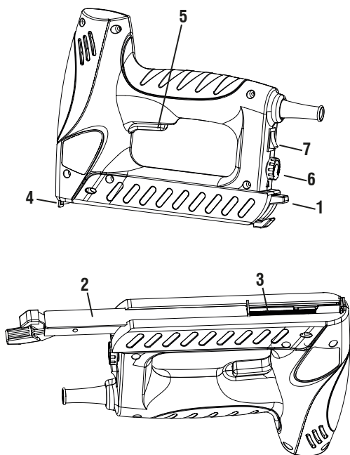
Fig. 1 – Componentes
