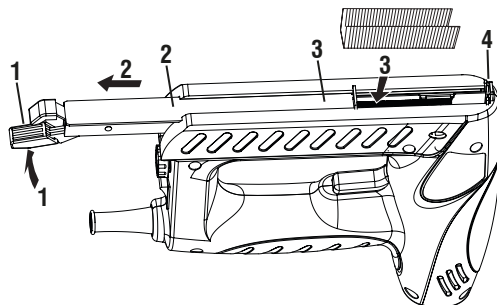
Fig. 2 – Carregando grampos/pinos
