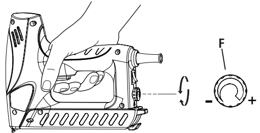
Fig. 5 – Control de impacto
