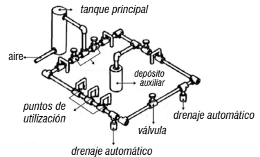
Fig. 1 – Red de aire comprimido
