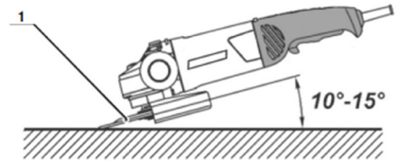
Fig. 8 – Ángulo correcto de esmerilado
