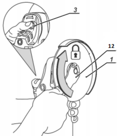
Fig. 6 – Montar el disco en la máquina
