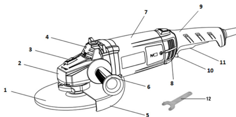
Fig. 1 – Componentes
