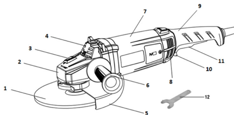
Fig. 1 – Componentes
