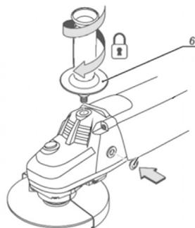
Fig. 2 – Ensamblar el mango auxiliar
