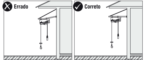
Fig. 10 - Instalar el soporte de modo que el equipo quede nivelado
