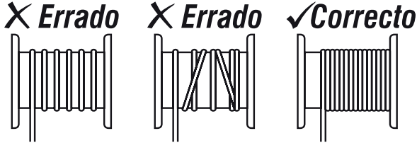
Fig. 16 – Enrollamiento
