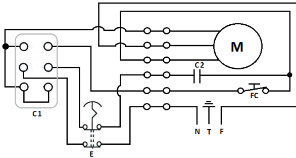
Fig. 17 – Esquema eléctrico para grúas 127 V~ y 220 V~
