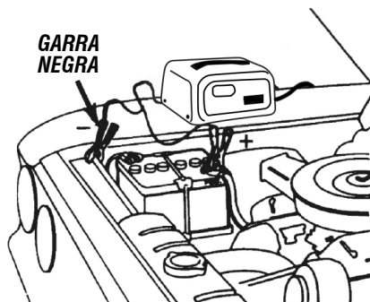
Fig. 3 – Carga con la batería en el vehículo
