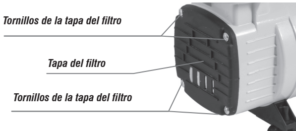
Figura 3 – Substitución del filtro
