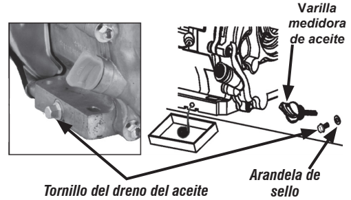
Fig. 8 – Cambio de aceite del cárter del motor
