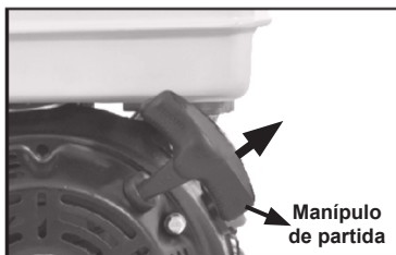
Fig. 7 – Manípulo do retrátil de partida
