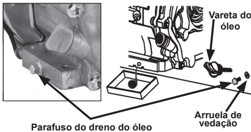
Fig. 8 – Troca de óleo do cárter do motor
