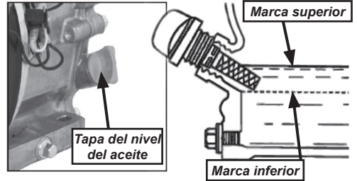
Fig. 2 – Aceite del motor
