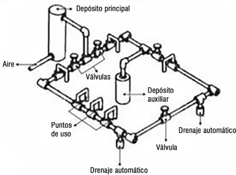
Fig. 1 – Red de aire comprimido
