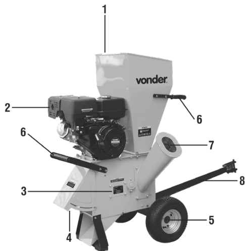
Fig. 1 – Componentes
