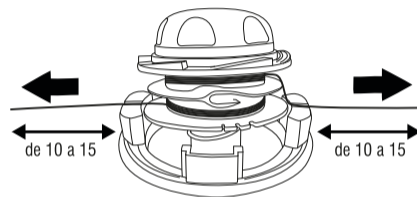
Fig. 3 – Comprimento do fio de nylon/Largo del hilo de nylon
