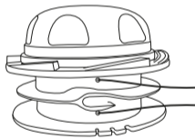
Fig. 2 – Passando o fio de nylon/Pasando el hilo de nylon.
