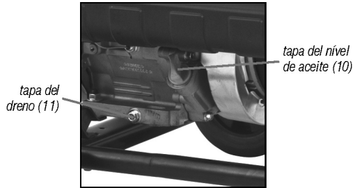
Fig. 7 – tapa del nivel de aceite (varilla)
