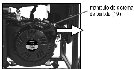
Fig. 19 – manípulo do sistema de partida manual
