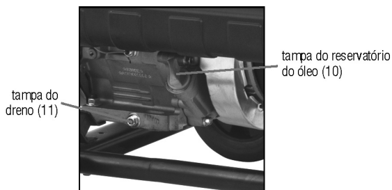
Fig. 7 – tampa de óleo (vareta)
