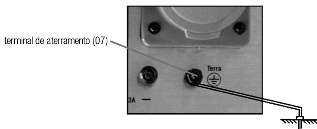
Fig. 15 – aterramento do gerador
