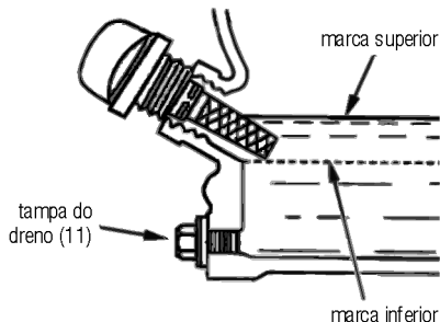
Fig. 8 – nível de óleo
