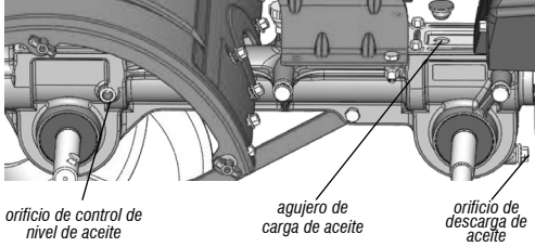
Fig. 9 – Posición para carga y descarga de aceite
