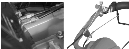
Fig. 5 – Ajuste dos cabos
