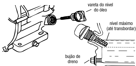
Fig. 8 – Nível de óleo
