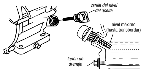
Fig. 8 – Nivel de aceite
