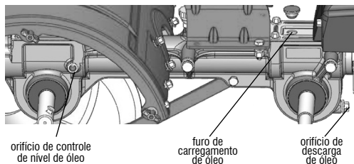
Fig. 9 – Posição para carga e descarga de óleo
