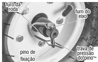
Fig. 6 – Modo roda livre
